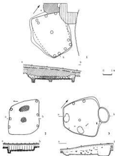
Рис. 4. Полуземлянки горизонта Боромля типа П\В: 1 – П\В1\аа (Боромля 2, сооружение 3); 2- П\В1\аб (Родной Край 3, сооружение 2); 3 – П\В1\аа (Боромля 2, сооружение 8).
