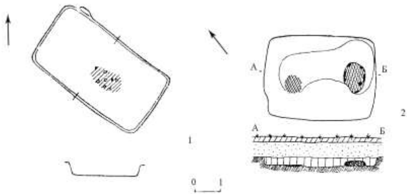
Рис. 2. Полуземлянки горизонта Боромля типа П\А: 1 – П\А 1\аа (Букреевка 2, сооружение 8), 2 – П\А 1\аб ( Родной Край 3, сооружение 1).
