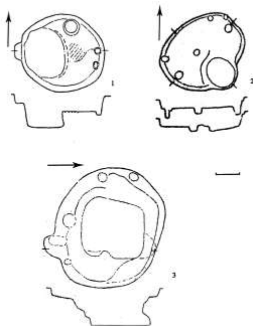
Рис. 1. Полуземлянки горизонта Боромля типа I: 1 – I\ 1а (Букреевка 2, сооружение 7), 2\ – I\1\ аб (Букреевка 2, сооружение 1), 3 – I\2аа (Букреевка 2, сооружение 4)
