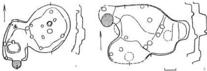
Рис.5. Полуземлянки горизонта Боромля типов: 1 - П1=аа + П\В\2аб (Букреевка 2, сооружение 2), 2 – П\А\1аб ( Букреевка 2, сооружение 5).
