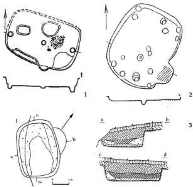
Рис. 3. Полуземлянки горизонта Боромля типа П\Б: 1- П\Б 1\аа (Букреевка 2, сооружение 9), 2 – П\Б 1\аб (Букреевка 2, сооружение 3); 3 – П\Б 1\бб (Боромля 2, сооружение 1).
